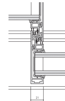
Interlock
