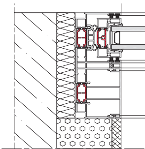
Jamb Detail
